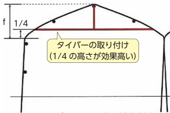
▲タイバーによる肩部の補強事例
