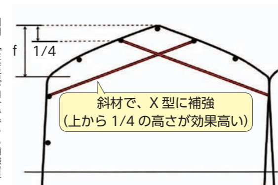
▲X型の斜材による肩部の補強事例
